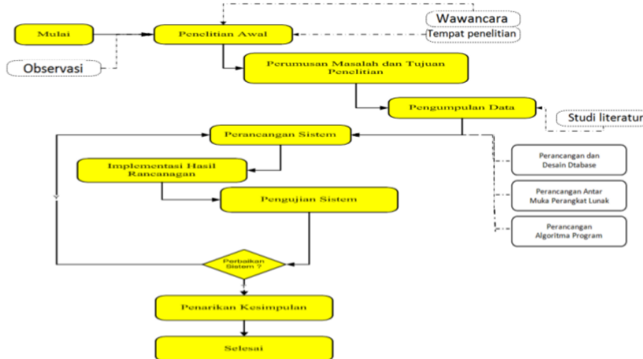
Gambar. 1. Tahapan Penelitian
