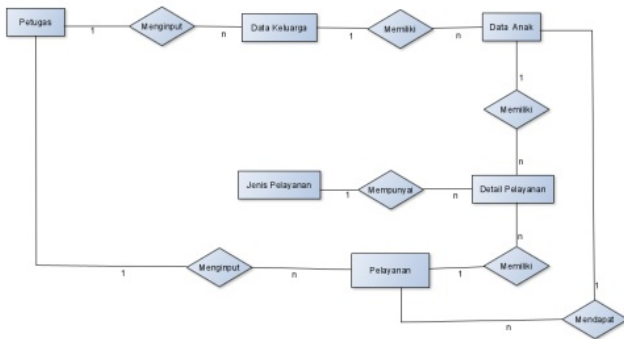
Gambar 8 ERD
