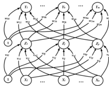
Gambar 2: Arsitektur Backpropagation
