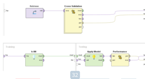
Gambar 1. Penerapan Algoritma K-NN dan k-Fold Cross Validation pada Tools Rapidminer
