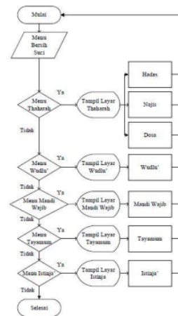
Gambar 2. Flowchart Menu Bersih Suci
