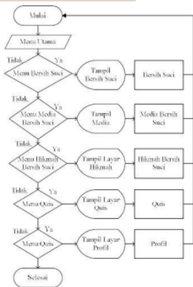
Gambar 1. Flowchart Menu Utama
