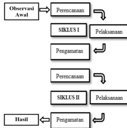
Gambar 1. Kerangka Penelitian
