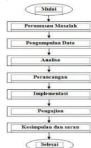
Gambar 3.1 Tahapan Penelitian
