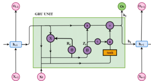
Gambar 2. Arsitektur GRU
