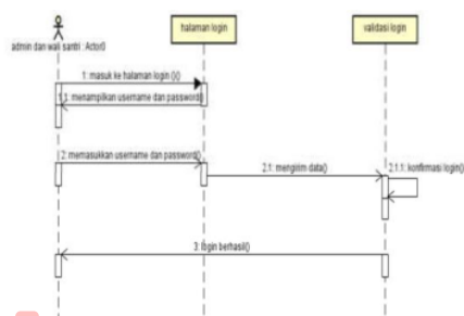
Gambar 4.6. sequence diagram melihat transaksi dan saldo
