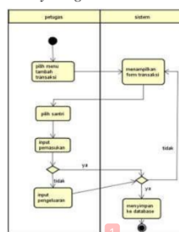
Gambar 4.4. activity diagram tambah transaksi
