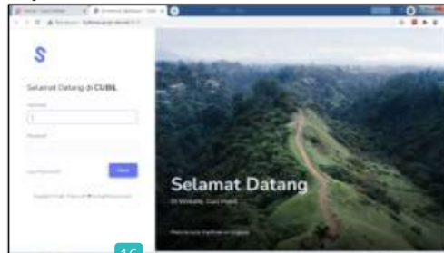
Gambar 3. Halaman Login
