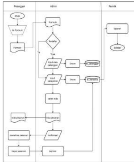
Gambar 2. Flowchart Sistem Kerja Setelah Perbaikan dengan Penerapan Sistem Informasi
