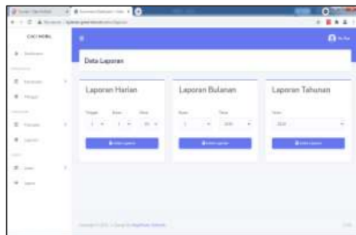
Gambar 8. Halaman Pelaporan
