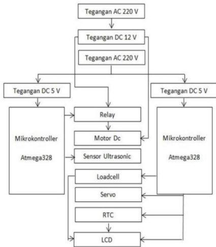
Gbr 6. Blok Diagram Keseluruhan Alat
