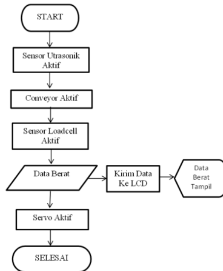
Gbr 10. Desain Sistem Kontrol Mesin Drop Box Telur
