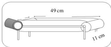
Gbr 7. Desain Sistem Conveyor Mesin Drop Box Telur
