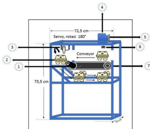
Gbr 5. Desain Casing Mesin Drop Box Telur (Tampak Samping)
