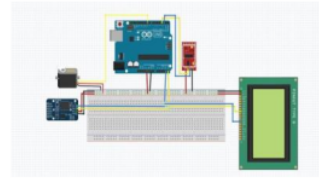
Gbr 8. Desain Sistem Elektrik dengan Arduino Uno
