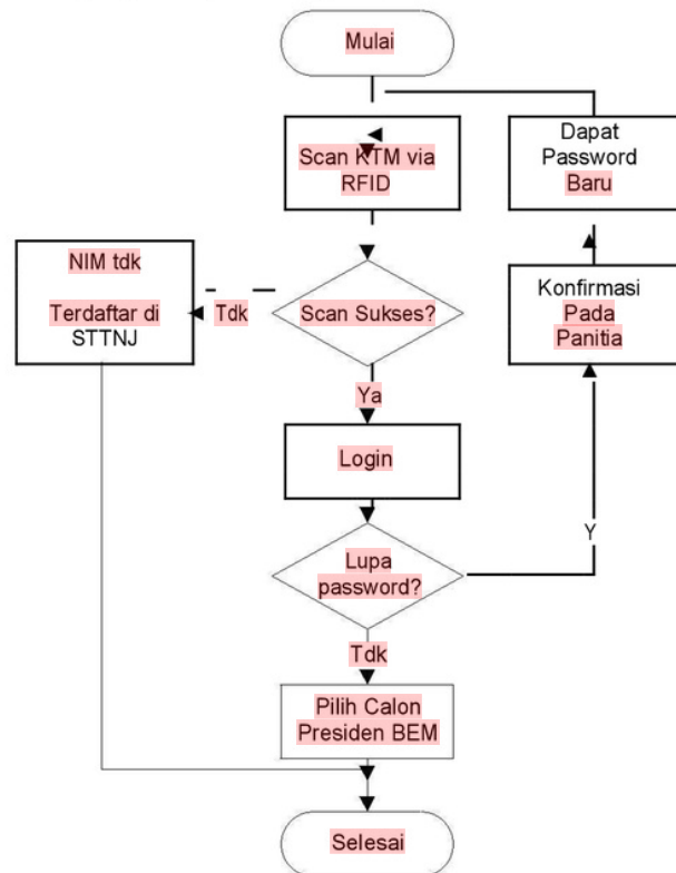
Gambar 1. Flowchart Pengoperasian Program Bagi Mahasiswa
