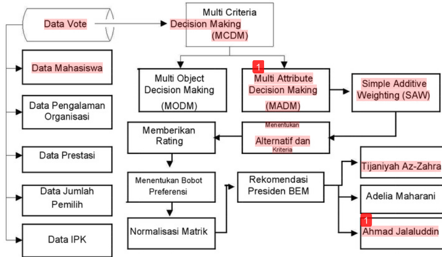
Gambar 2. Konsep Solusi Permasalahan
