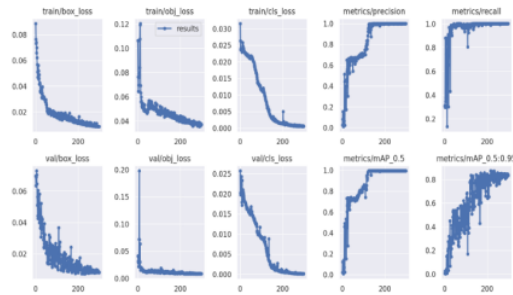
Gambar 12. Hasil Training Menggunakan YOLOv5s6
