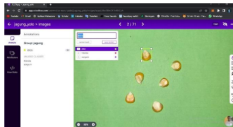
Gambar 3. Anotasi Data
