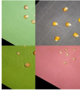
Gambar 7. Hasil Augmentasi
