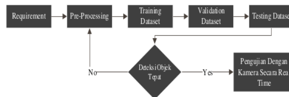
Gambar 1. Tahapan Penelitian
