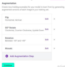
Gambar 6. Proses Augmentasi
