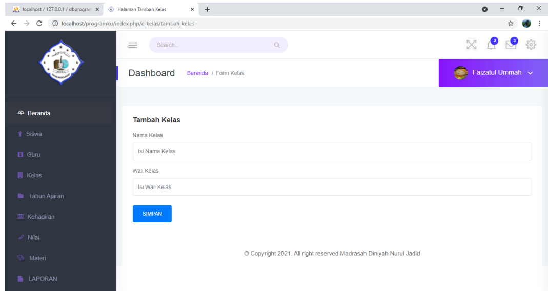
Gambar 4.28 Halaman Tambah Kelas
