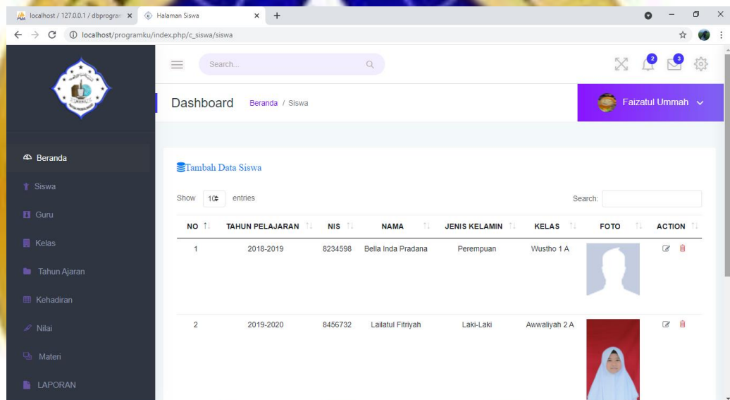
Gambar 4.23 Halaman Siswa
