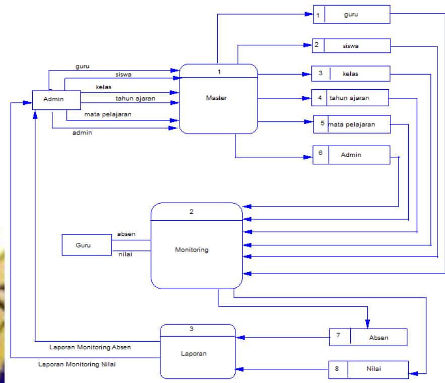
Gambar 4.6 DFD Level 1
