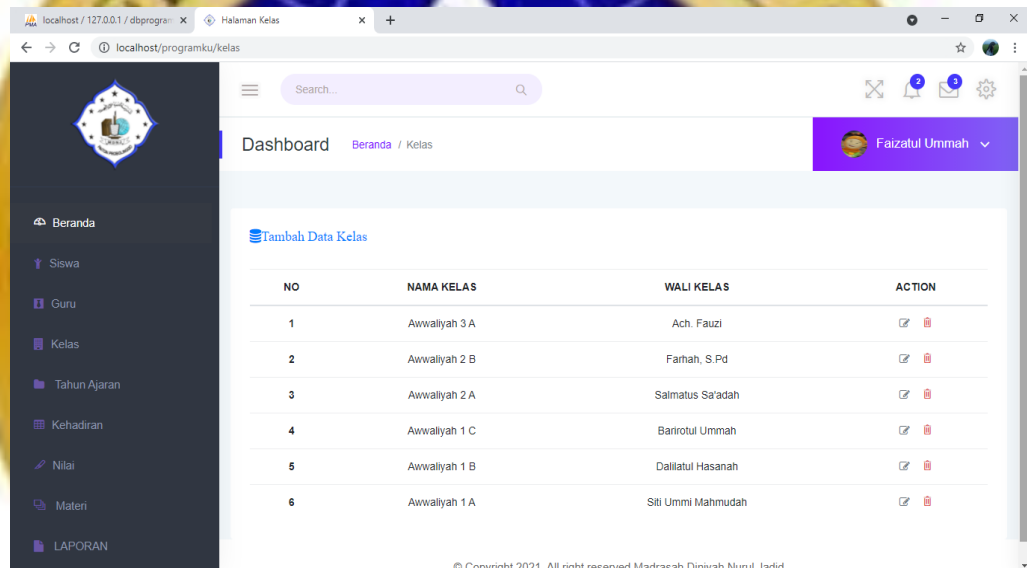
Gambar 4.27 Halaman Kelas
