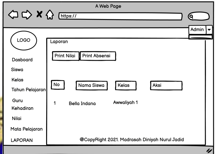
Gambar 4.20 Desain Monitoing
