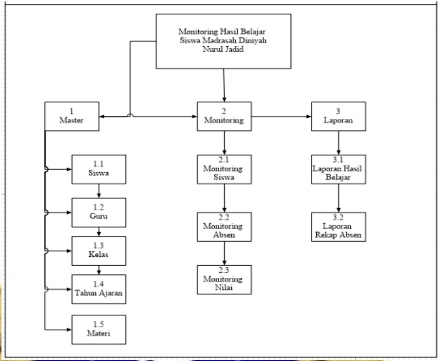
Gambar 4.5 Bagan Berjenjang
