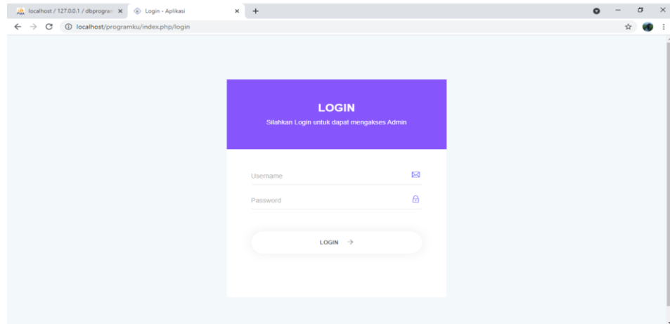
Gambar 4.21 Halaman Login
