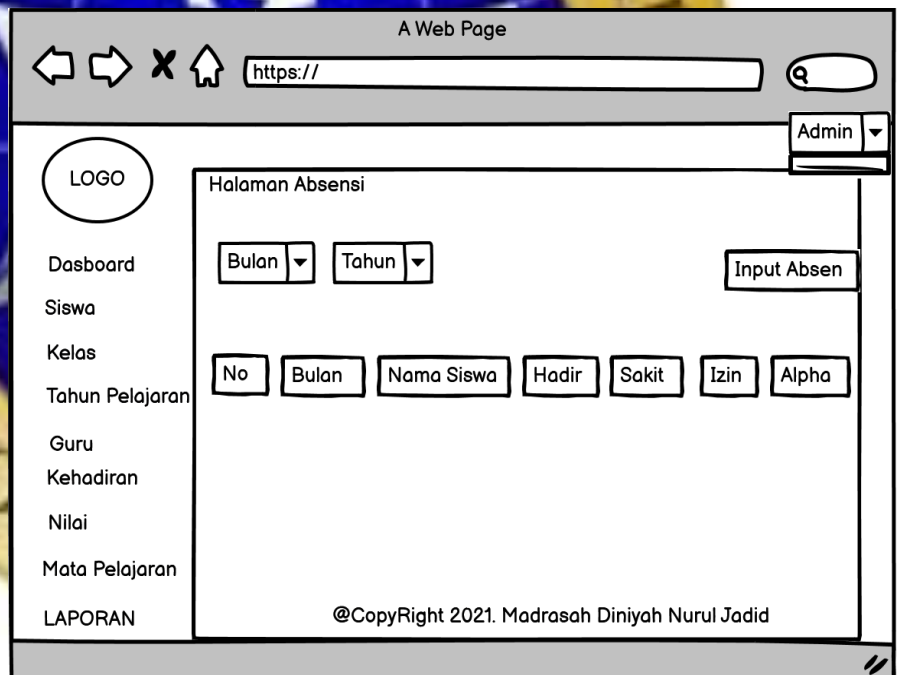
Gambar 4.15 Desain Halaman Absen
