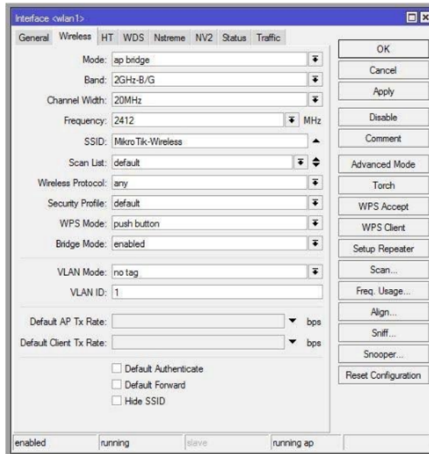
Gambar 16. Setting wlan1
