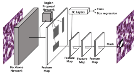
Gambar 2. Arsitektur Mask R-CNN
